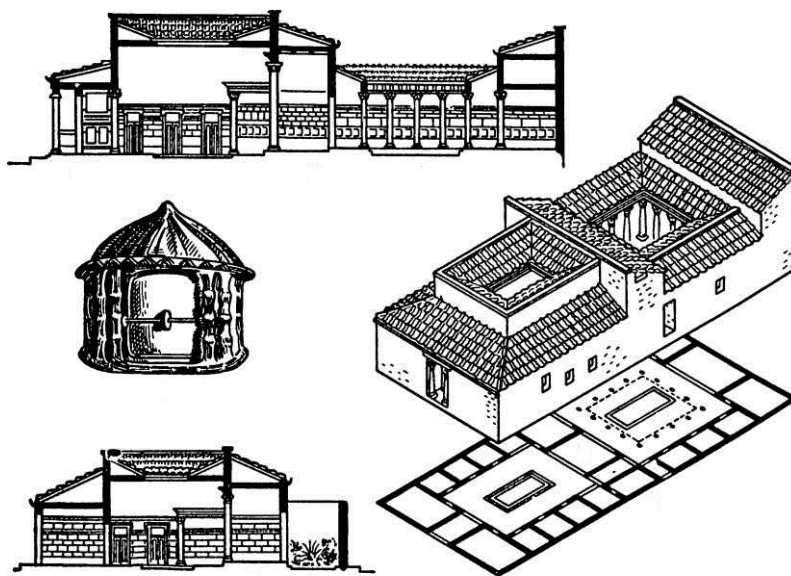
Рис. 1. План, разрезы и общий вид атриумно-перистильного дома
