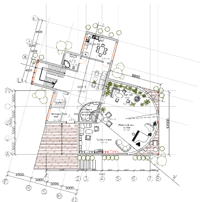
Рис. 2. Общий вид и план дома «Квартет»
